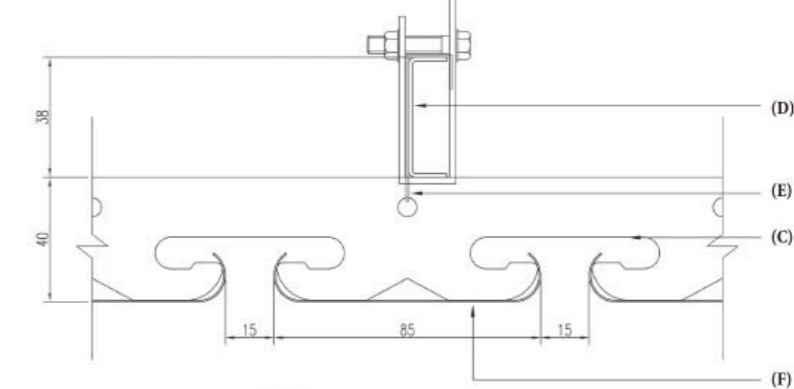
Section Drawing / 正面节点图
